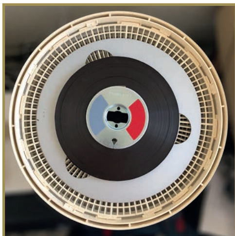
A gauche : Traitement d'une bande Ampex de 1980 atteinte de "Sticky Shed Syndrome" : Chauffage dans un four spécial avec contrôle de température, afin d'en extraire l'humidité et ainsi éviter qu'elle ne colle et perde son oxyde sur les guides et les têtes de lecture.
